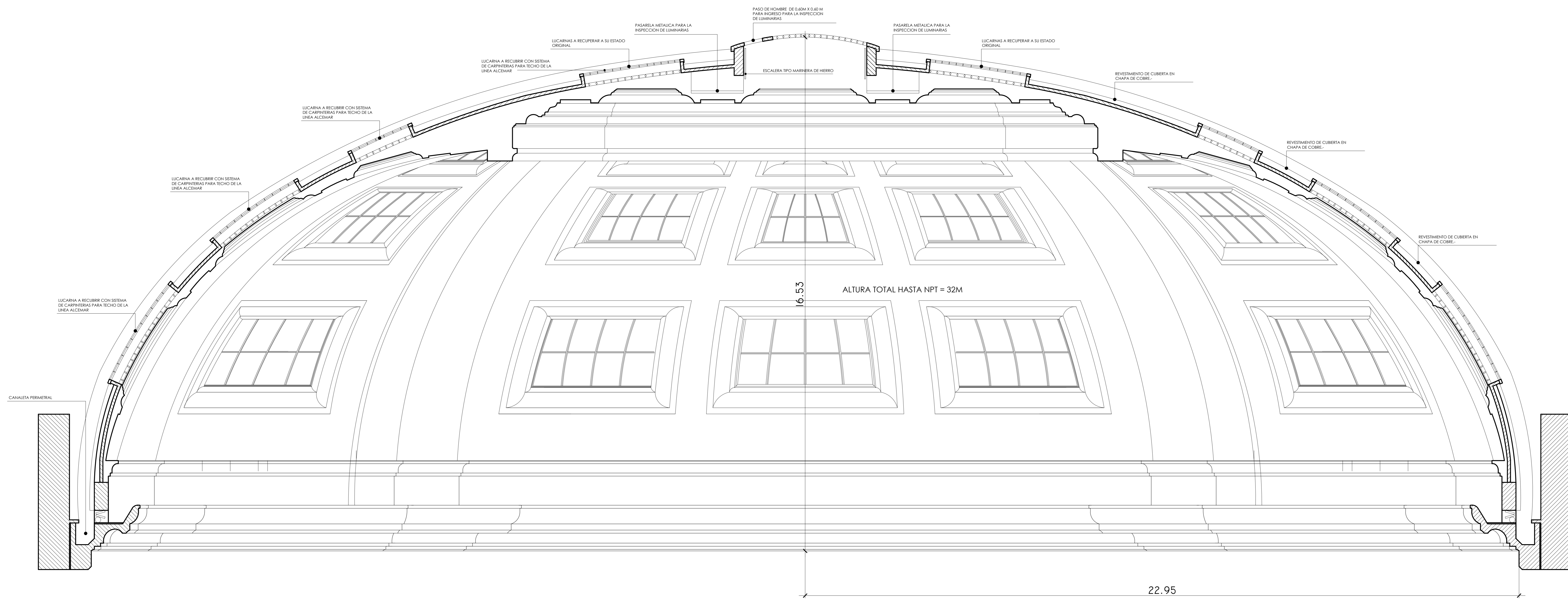
CORTE A-B
